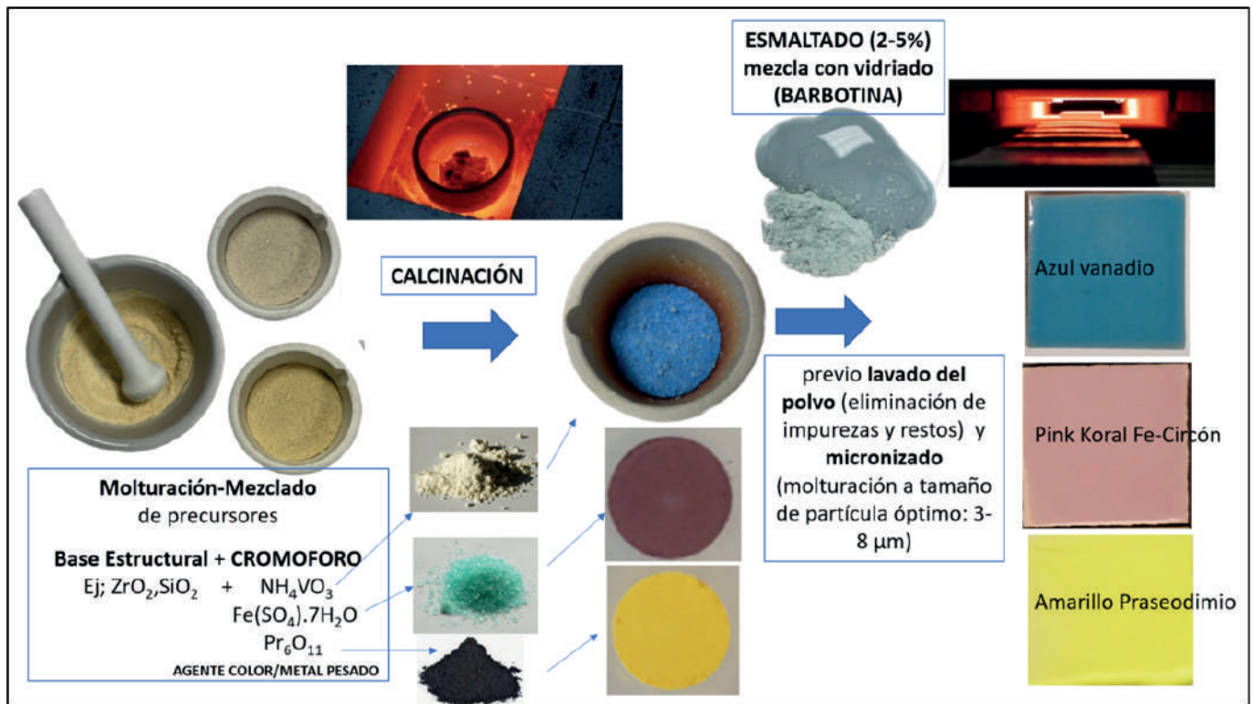
Figura 3. Proceso general de la producción de la familia del circonio o silicato de circonio.
